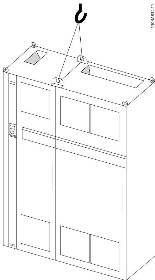
Illustration 3.4 建议起吊方法，机架规格 F1。
