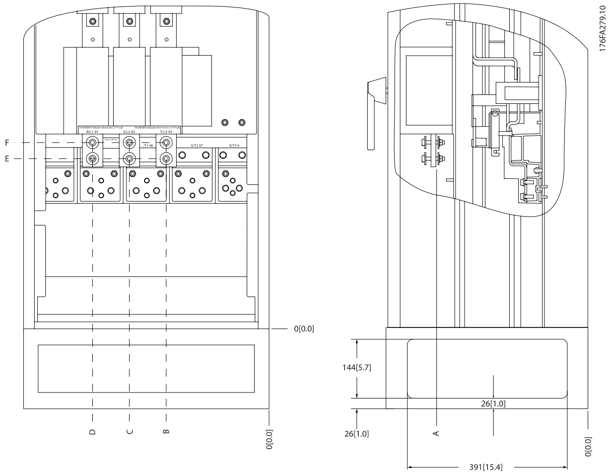
Illustration 3.18 IIP21 ( NEMA 类型 1 ) 和 IP54 ( NEMA 类型 12 ) 机箱 的断路开关的电源接头位置
