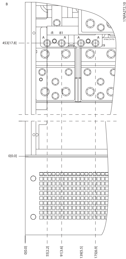
Illustration 3.17 IP21 (NEMA 类型 1) 和 IP54 (NEMA 类型 12) 机箱 的电源接头位置 ( B 处的局部视图 )
