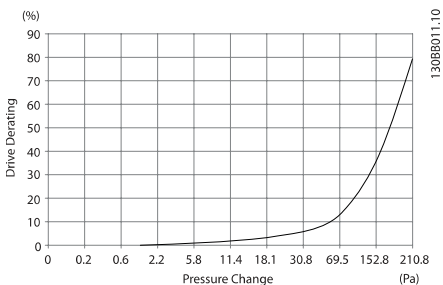
Illustration 3.32 E 机架 的降容与 压力变化 ( 大风扇 ) P355T5-P450T5 和 P630T7-P560T7
