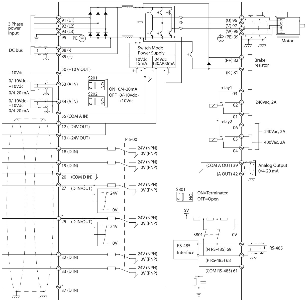
Illustration 4.17 图中显示了不带选件时的所有电气端子。
