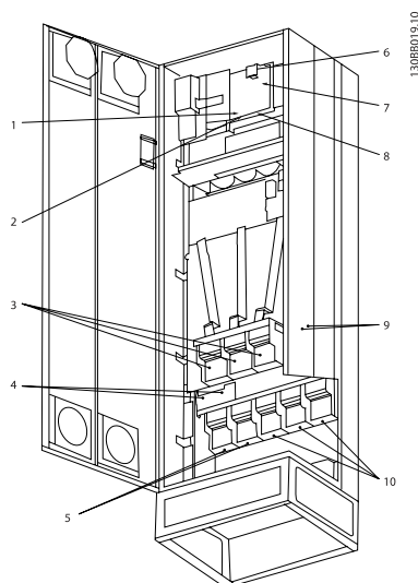
Illustration 4.7 紧凑型 IP 21 ( NEMA 1 ) 和 IP 54 ( NEMA 12 ) , 机架规格 E1
