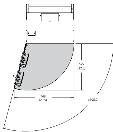
Illustration 3.9 IP21/IP54 机箱类型，机架规格 E1 的前方空间。
