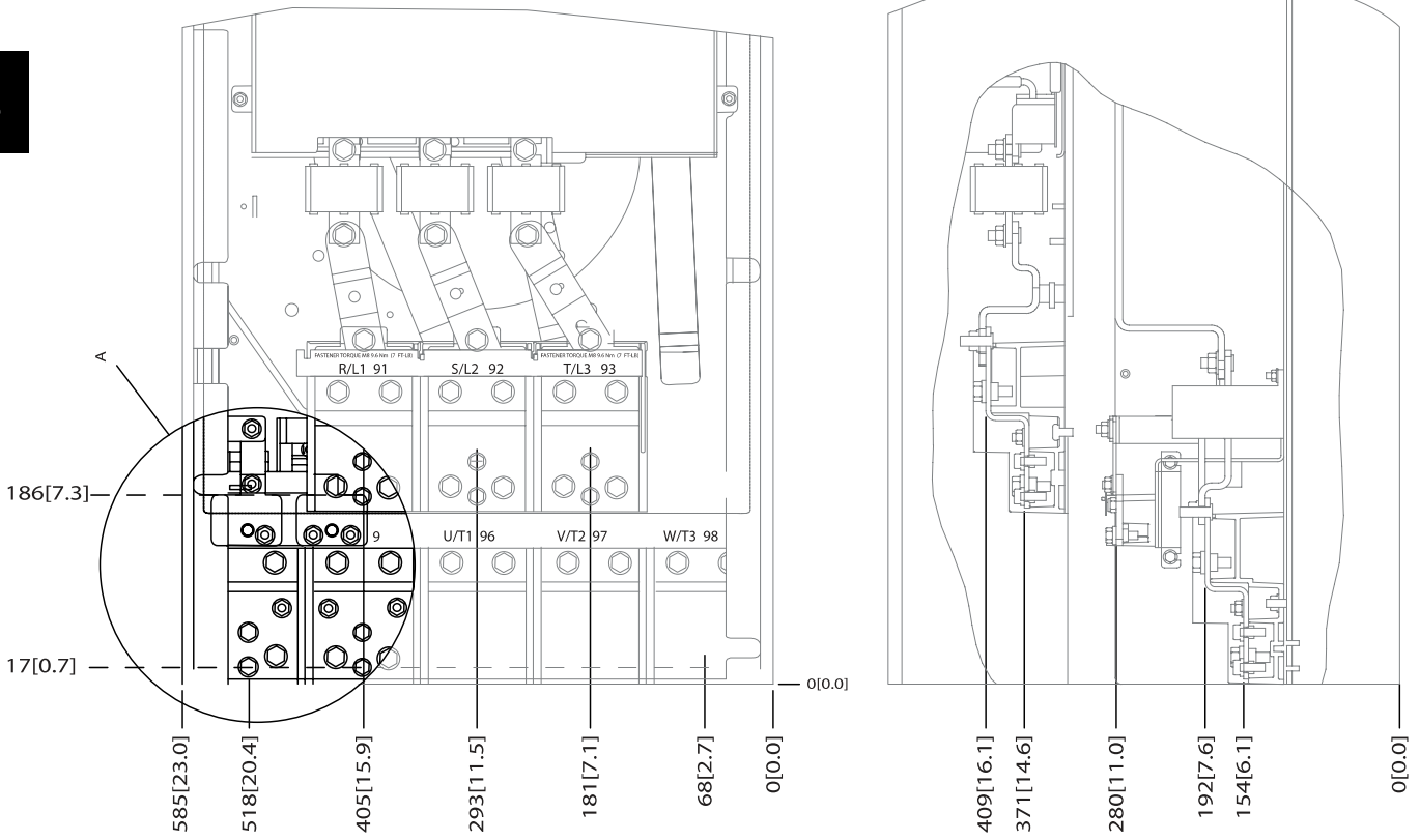
Illustration 3.19 IP00 机箱 的电源接头位置
