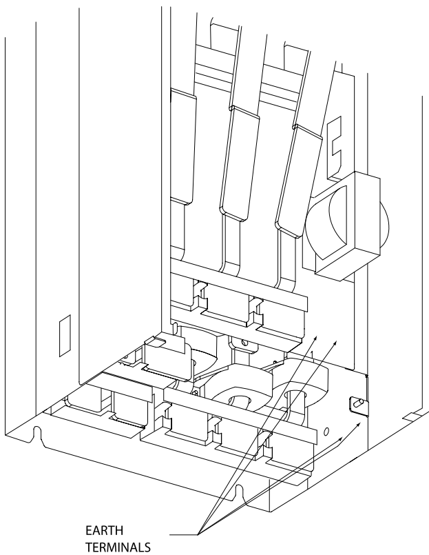
Illustration 4.5 IP00, 机架规格 D 的接地端子的位置
