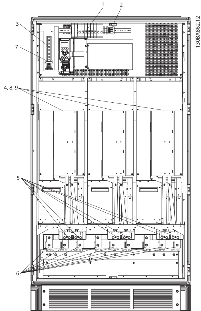
Illustration 4.12 逆变器机柜，机架规格 F2 和 F4
