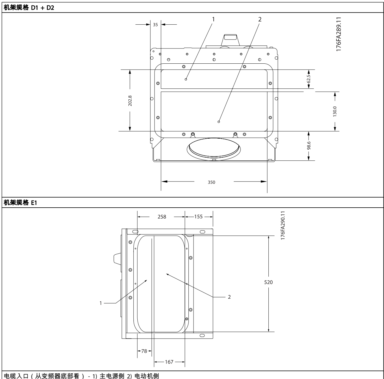
Illustration 3.35 正确安装密封板的示例。
