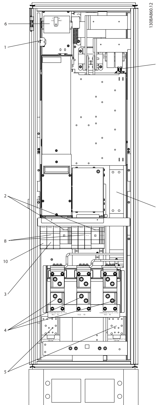
Illustration 4.10 整流器机柜，机架规格 F1、F2、F3 和 F4
