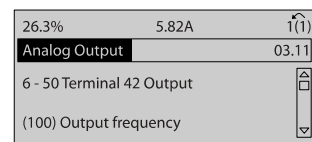
Illustration 6.7 步骤 6: 选择参数 6-50。按 [OK] (确定)。
