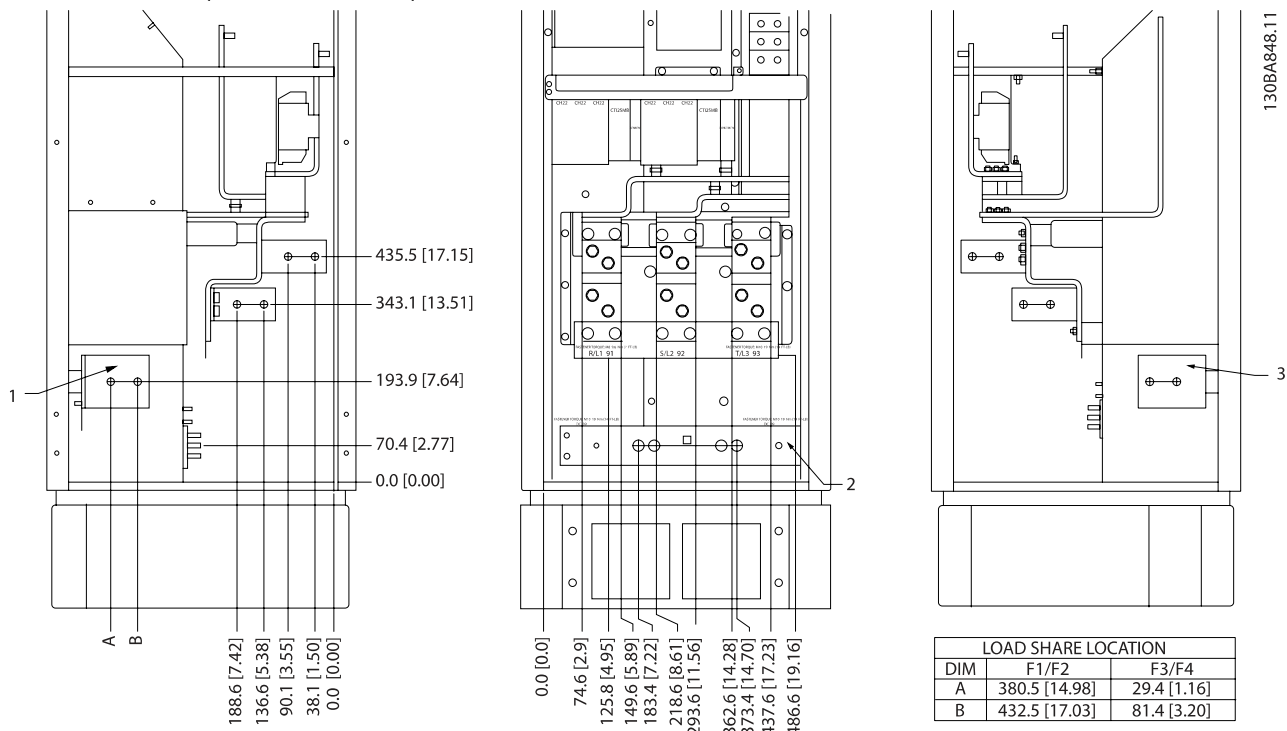
Illustration 3.27 端子位置 - 整流器 (左、正和右视图)。密封板比 0 平面低 42 mm。
