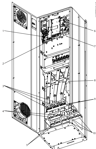
Illustration 4.1 紧凑型 IP 21 (NEMA 1) 和 IP 54 (NEMA 12), 机架规格 D1
