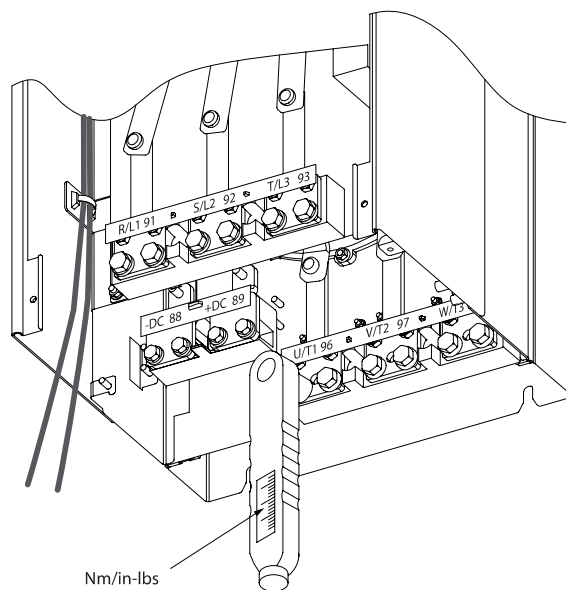
Illustration 4.14 总是使用转矩扳手来拧紧螺栓。
