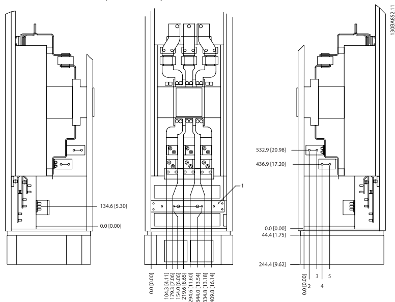
Illustration 3.29 端子位置 - 带断路器/模壳开关的选件机柜 ( 左、正和右视图 )。密封板比 0 平面低 42 mm。
