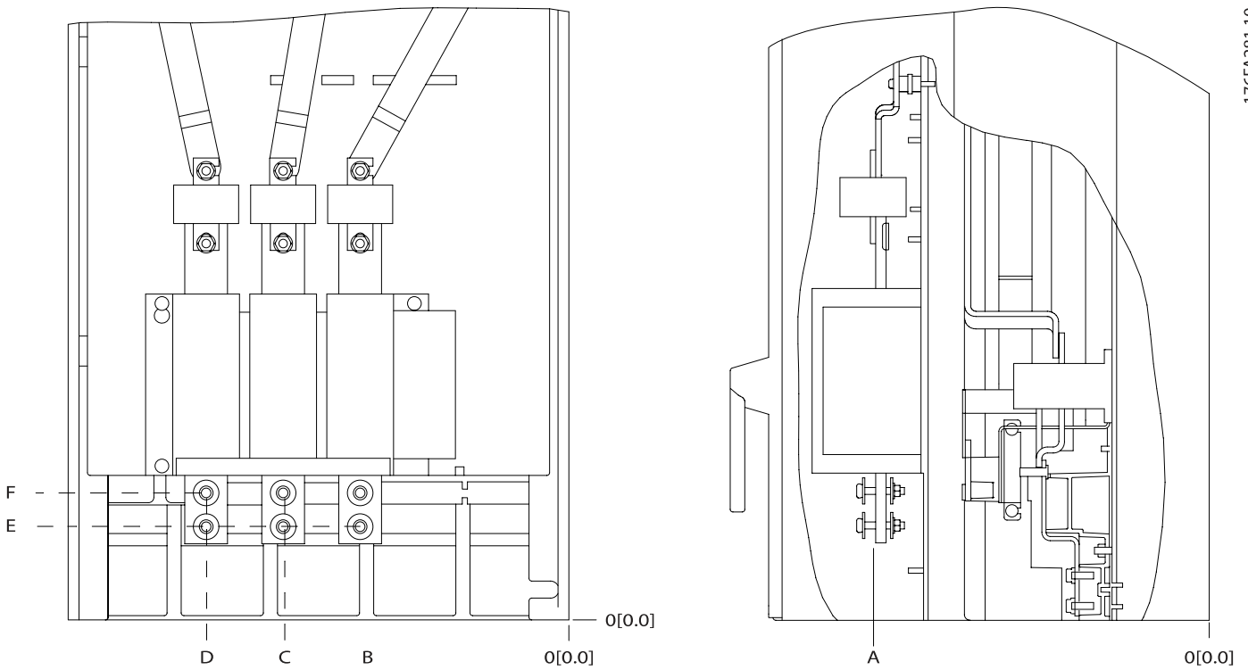
Illustration 3.21 IP00 机箱的断路开关的电源接头位置
