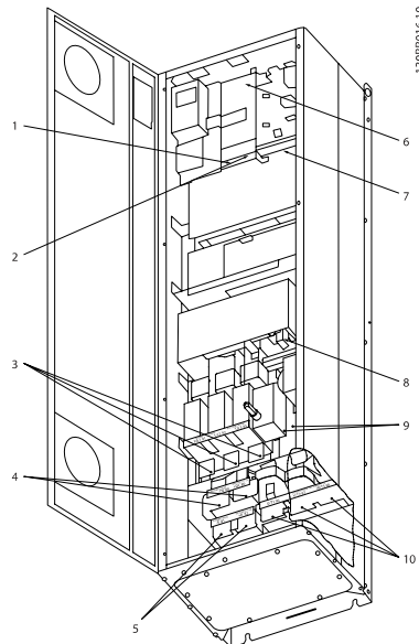
Illustration 4.2 紧凑型 IP 21 (NEMA 1) 和 IP 54 (NEMA 12), 带断路器、保险和射频干扰滤波器, 机架规格 D2
