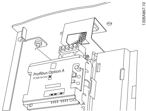
Illustration 4.16 从顶部连接现场总线。
