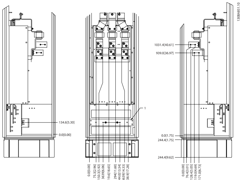
Illustration 3.28 端子位置 - 选件机柜 (左、正和右视图)。密封板比 0 平面低 42 mm。
