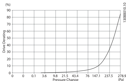
Illustration 3.31 E 机架 的降容与 压力变化 ( 小风扇 ), P315T5 和 P450T7-P500T7
