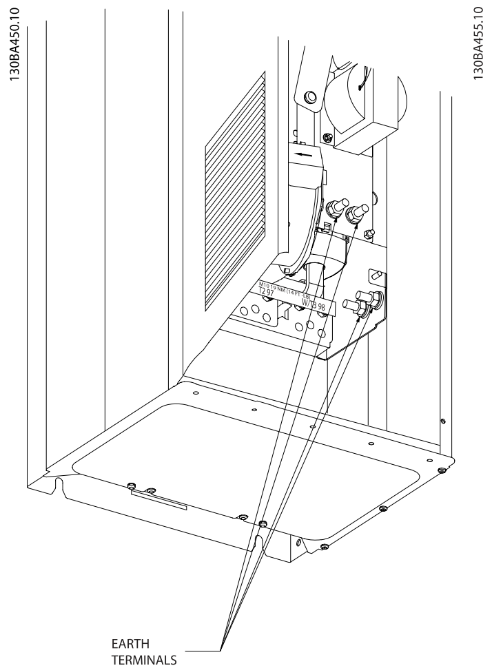
Illustration 4.6 IP21 ( NEMA 类型 1 ) 和 IP54 ( NEMA 类型 12 ) 的接地端子位置
