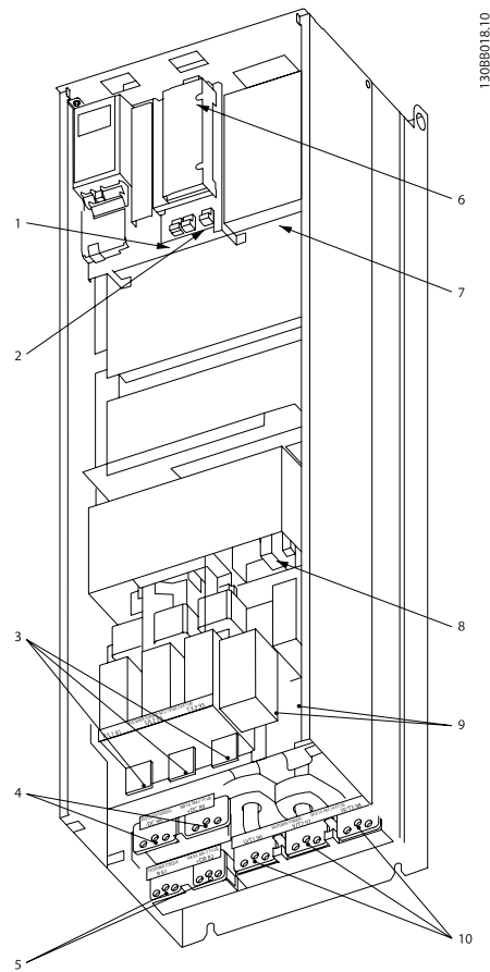
Illustration 4.4 紧凑型 IP 00 ( 机架式 ), 带断路器、保险装置和射频干扰滤波器, 机架规格 D4
