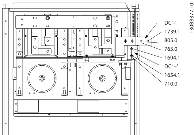
Illustration 3.24 端子位置 - Regen 端子 - F1 和 F3
