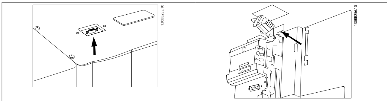
Illustration 4.16 从顶部连接现场总线。
