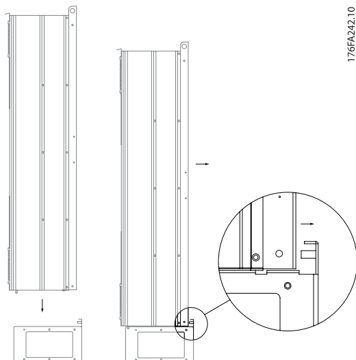
Illustration 3.40 将变频器安装到底座上。
