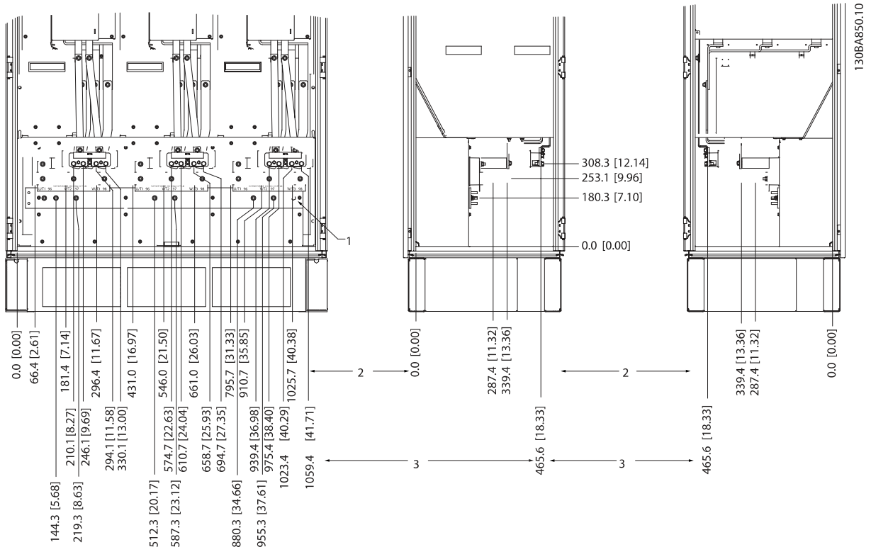
Illustration 3.25 端子位置 - 逆变器机柜 - F2 和 F4 ( 正、左和右视图 )。密封板比 0 平面低 42 mm。
