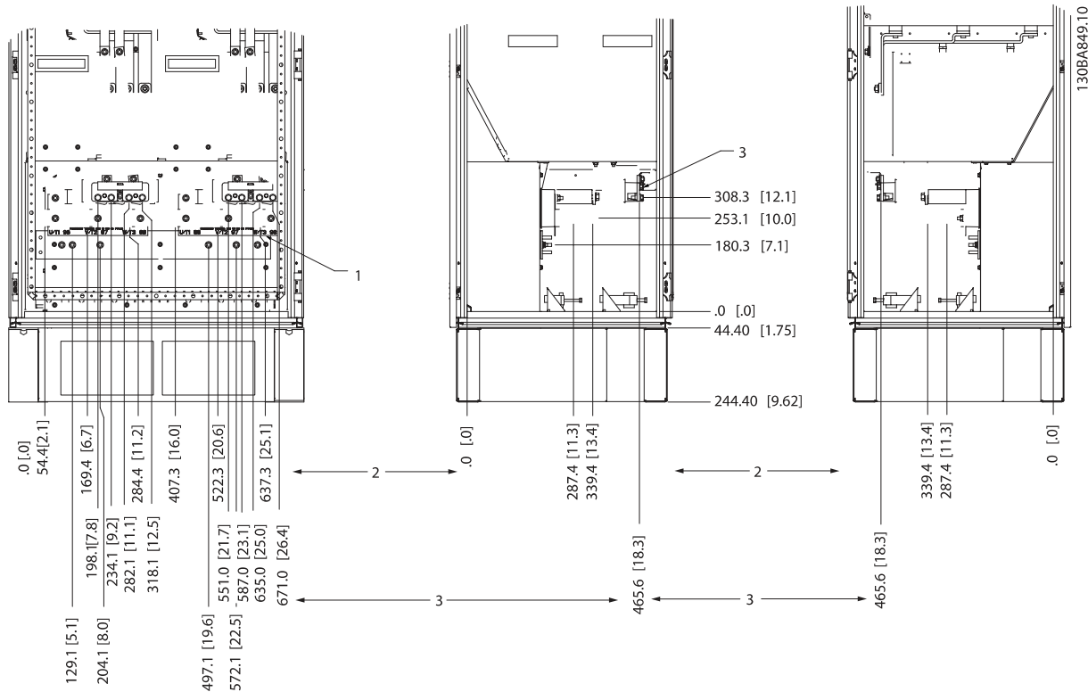
Illustration 3.23 端子位置 - 逆变器机柜 - F1 和 F3 ( 正、左和右视图 )。密封板比 0 平面低 42 mm。
