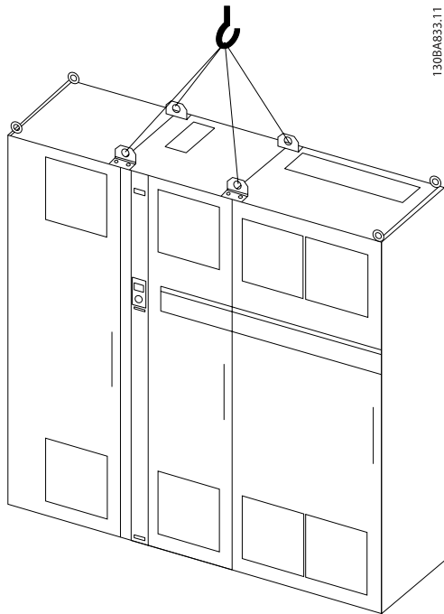
Illustration 3.6 建议起吊方法，机架规格 F3。
