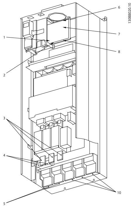
Illustration 4.8 紧凑型 IP 00 ( 机架式 ), 带断路器、保险装置和射频干扰滤波器, 机架规格 E2
