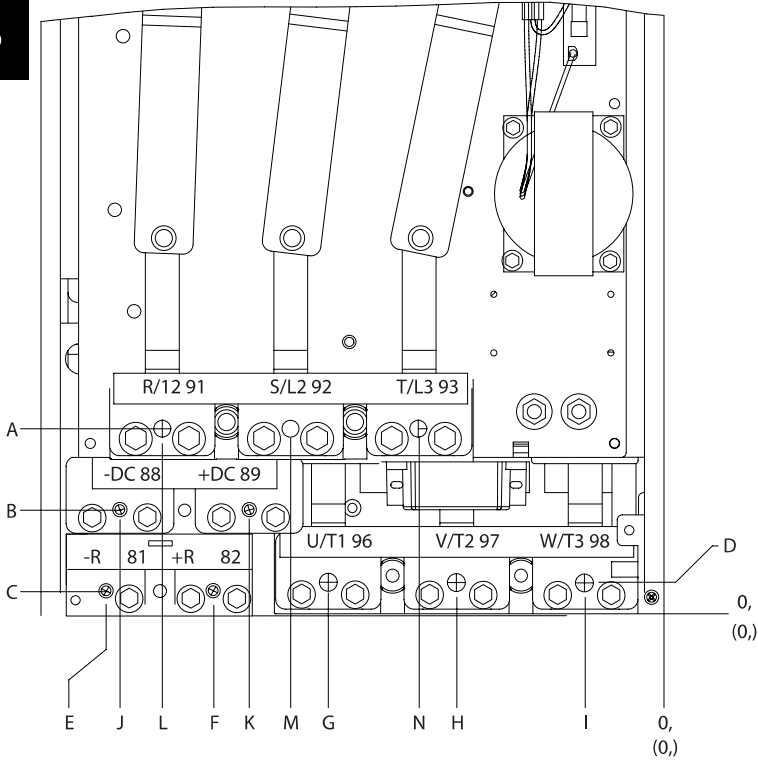
Illustration 3.14 电源连接的位置，机架规格 D3 和 D4
