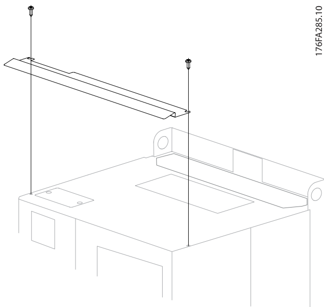
Illustration 3.37 遮护板安装。
