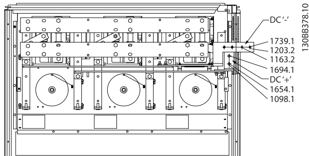
Illustration 3.26 端子位置 - Regen 端子 - F2 和 F4
