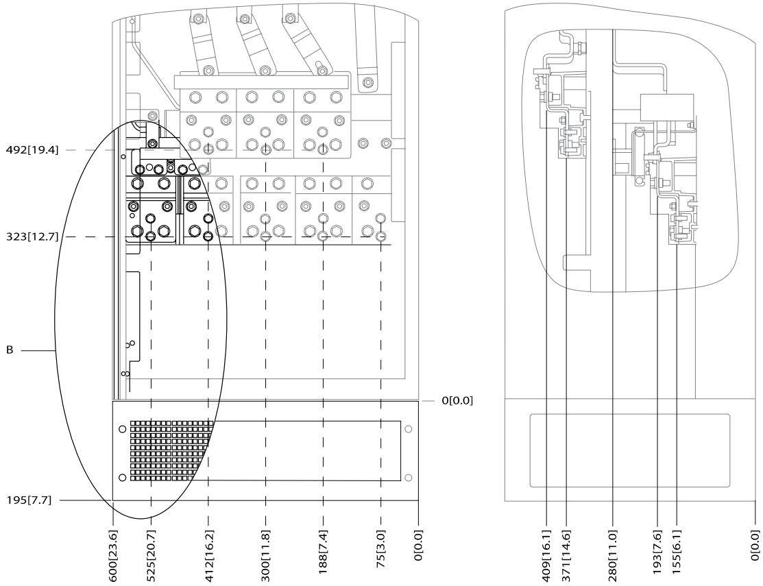
Illustration 3.16 IP21 (NEMA 类型 1) 和 IP54 (NEMA 类型 12) 机箱的电源接头位置
