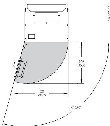
Illustration 3.8 IP21/IP54 机箱类型，机架规格 D1 和 D2 的前方空间。
