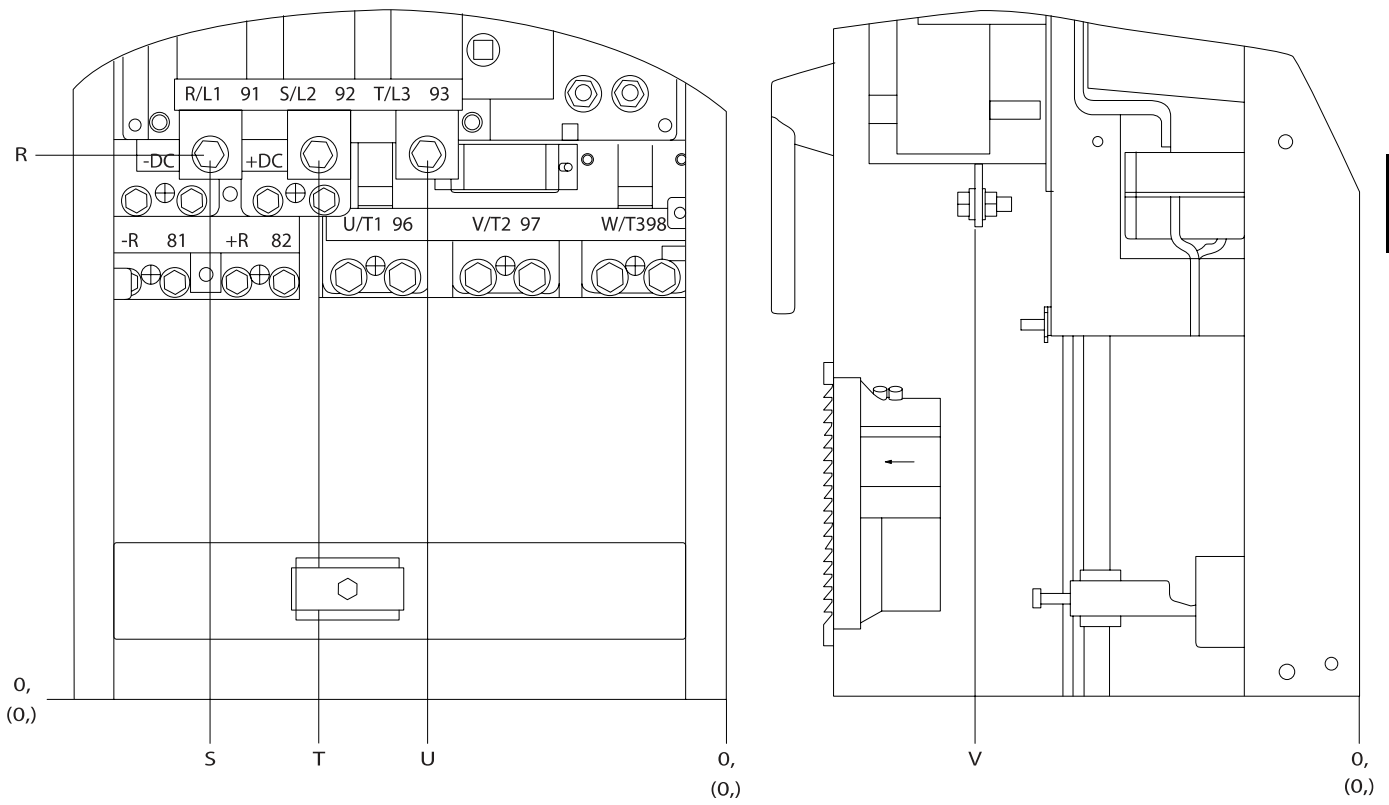
Illustration 3.15 电源连接 ( 带断路器 ) 的位置，机架规格 D1 和 D2
