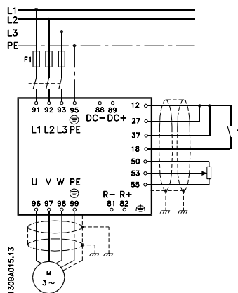
Illustration 3.1 此图显示了基本安装，其中包括主电源、电动机、启动/停止键以及用于调整速度的电位计。
