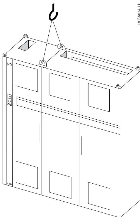
Illustration 3.5 建议起吊方法，机架规格 F2。
