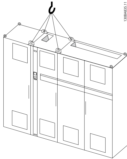
Illustration 3.7 建议起吊方法，机架规格 F4。
