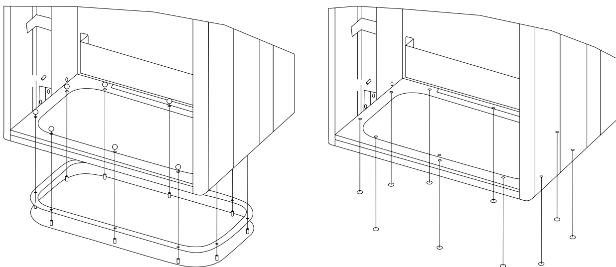
Illustration 3.36 底板安装，机架规格 E1。
